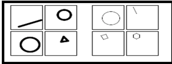
Fig. 2.5: Bongo CAPTCHA
