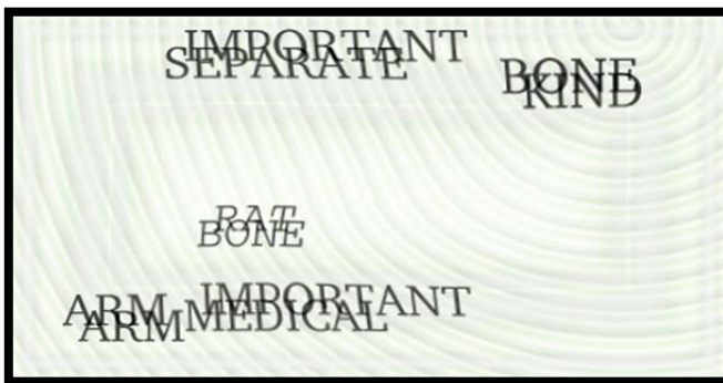
Fig. 2.1: Gimpy CAPTCHA
